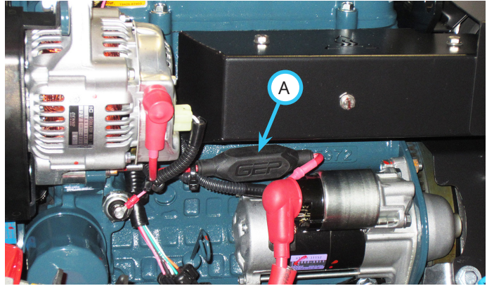
Bezpieczniki silnika
