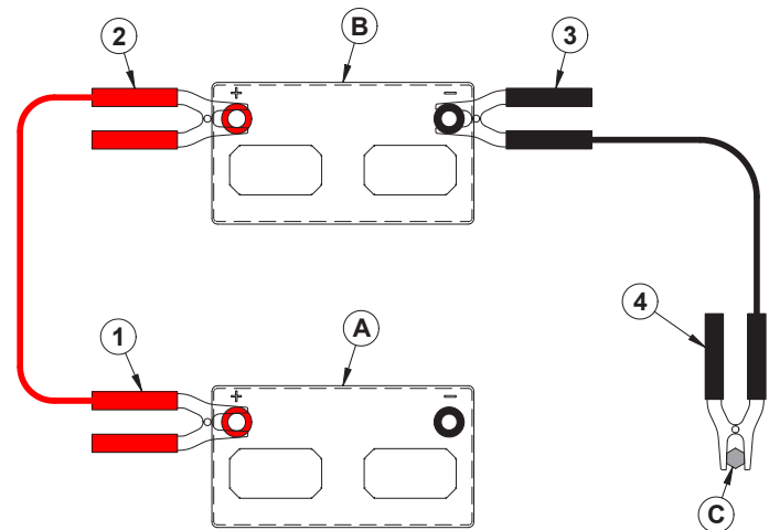
A. Akumulator rozładowany B. Akumulator wspomagający C. Kołek uziemiający
