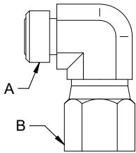
25.FF6500-(xx)-(xx) Fitting
