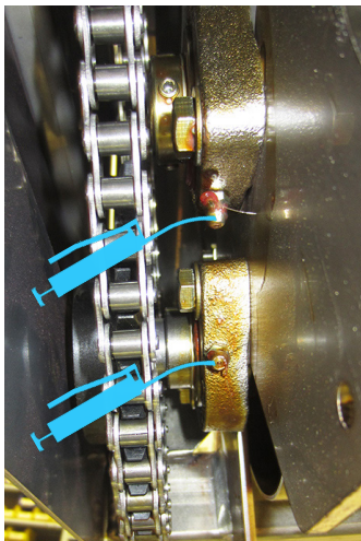
Levá ložiska
