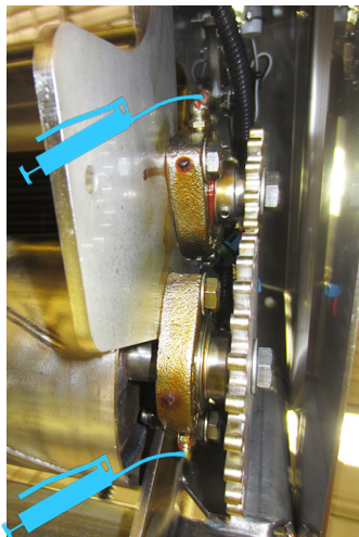
Pravá ložiska
